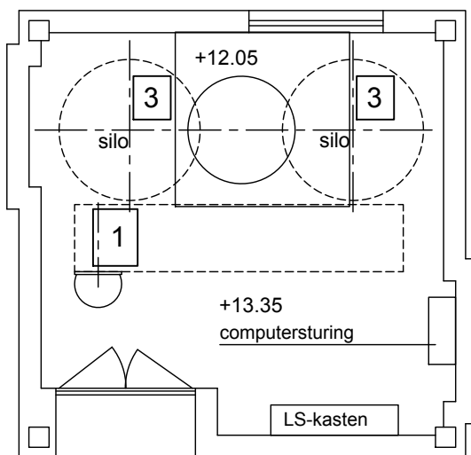
Gelijkvloers (niv 13.35)
