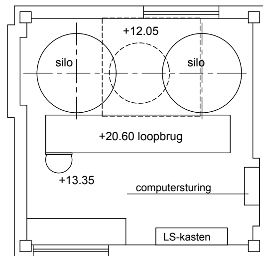
loopbrug (niv 20.60)
