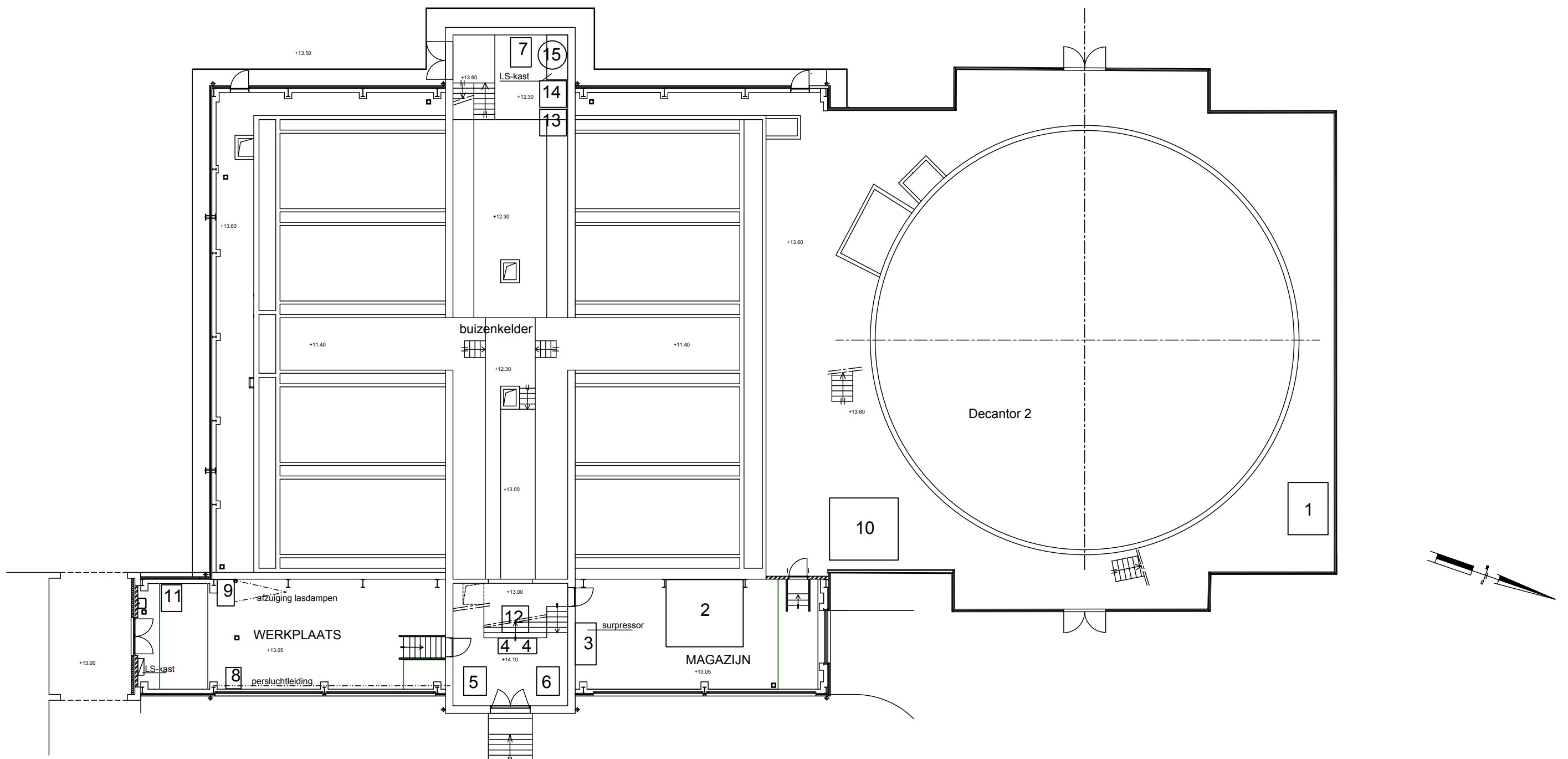
Decantor 2 - gelijkvloers/buizenkelder
