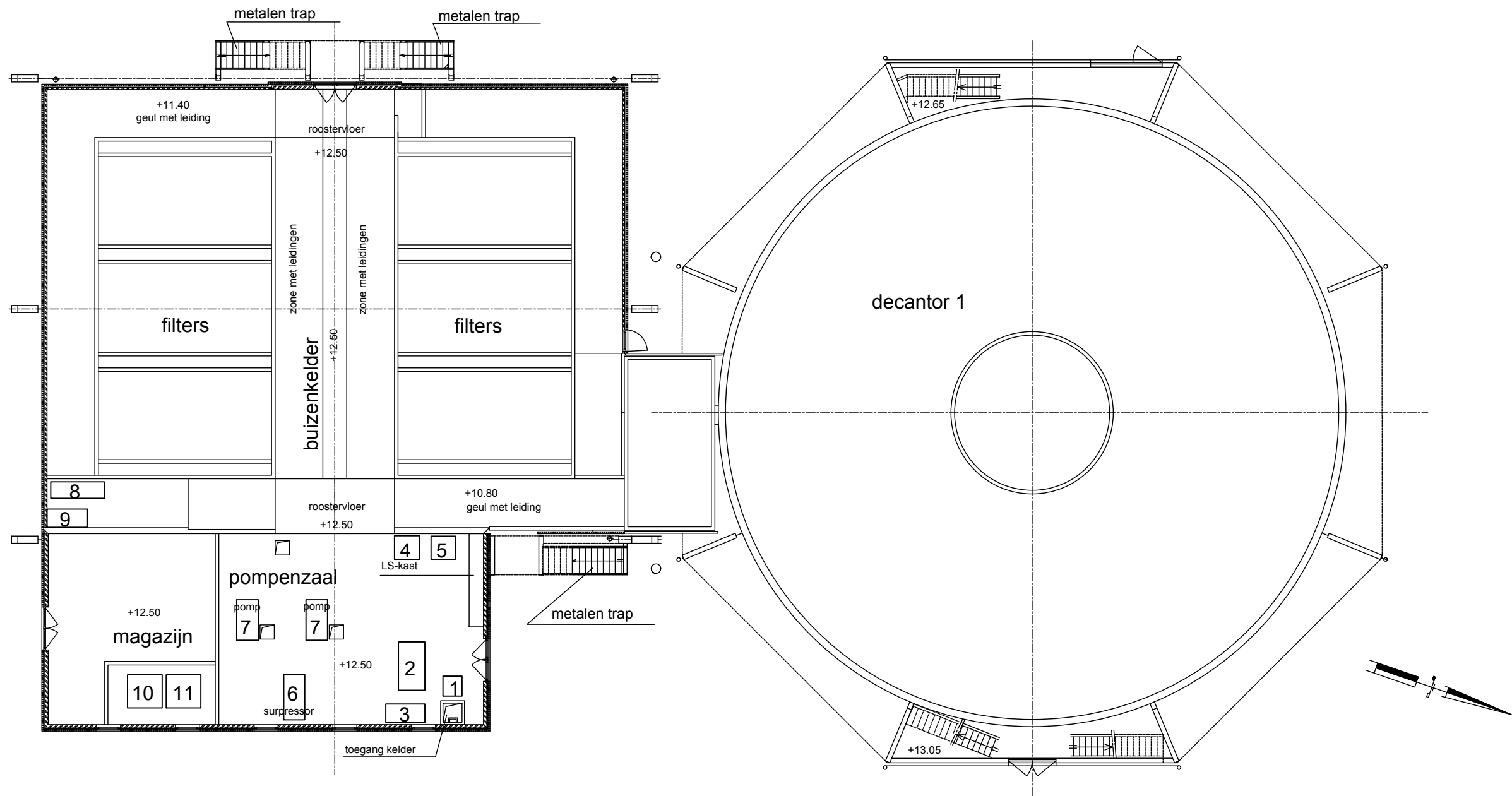
Filters en decantor 1 - gelijkvloers/buizenkelder
