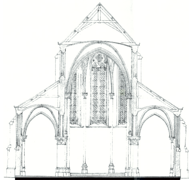
DWARSDOORSNEDE
