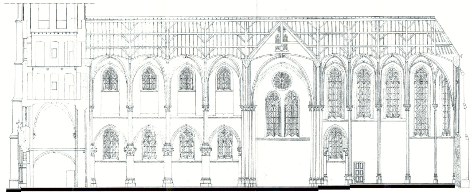
LANGSDOORSNEDE
