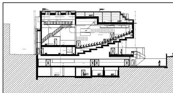
doorsnede van het nieuwe cultuurcentrum
